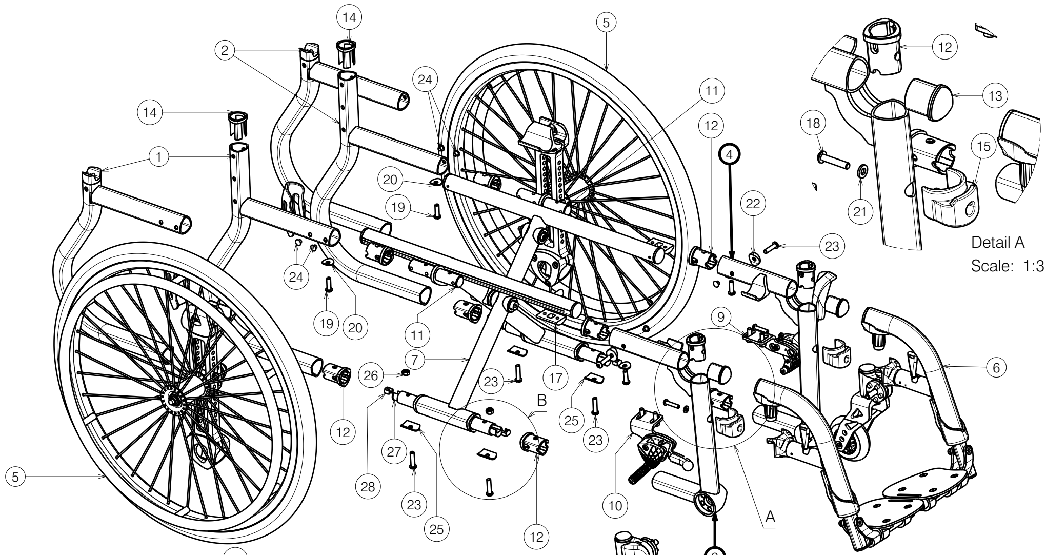
Isometric view Scale: 1:6
